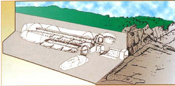
VISTA EN PERSPECTIVA D'UN HIPOGEU DE CALA SANT VICENÇ (MALLORCA) (SEGONS ROSSELLÓ BORDOY, PLANTALAMOR I MURILLO, RETOCADA PER SYLVIA GILI)
