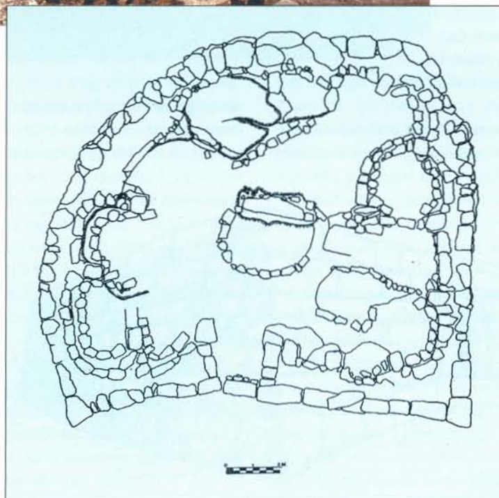
PLANTA DEL RECINTE DE TAULA DE TORRALBA D'EN SALORD (ALAIOR, MENORCA) (SEGONS M. FERNÁNDEZ-MIRANDA)
